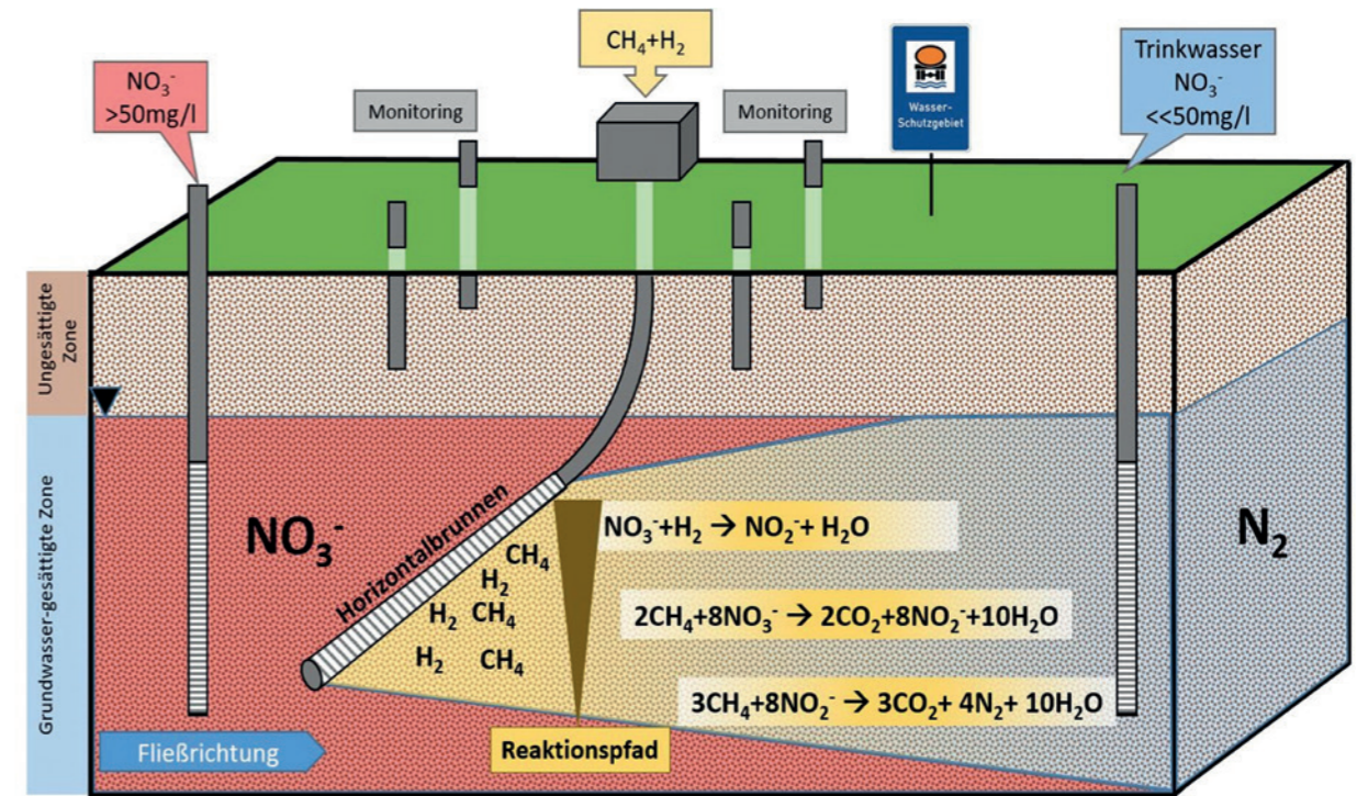
Schematische Darstellung eines Porengrundwasserleiters mit niedergebrachter Bohrung und Ausbringung der reaktiven Gase zur Stimulation der Denitrifikation über eine Horizontalbohrung. (Quelle: NitratLurch)
